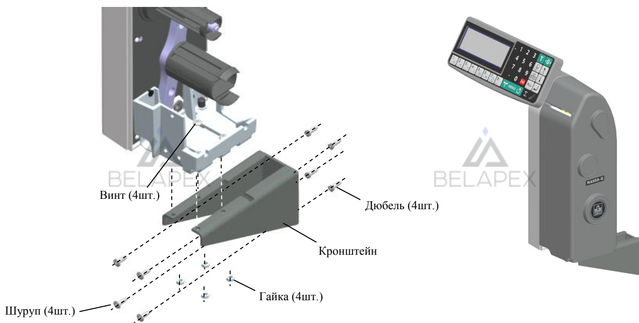
Рис. 2.5 – Крепление терминалов на стене
