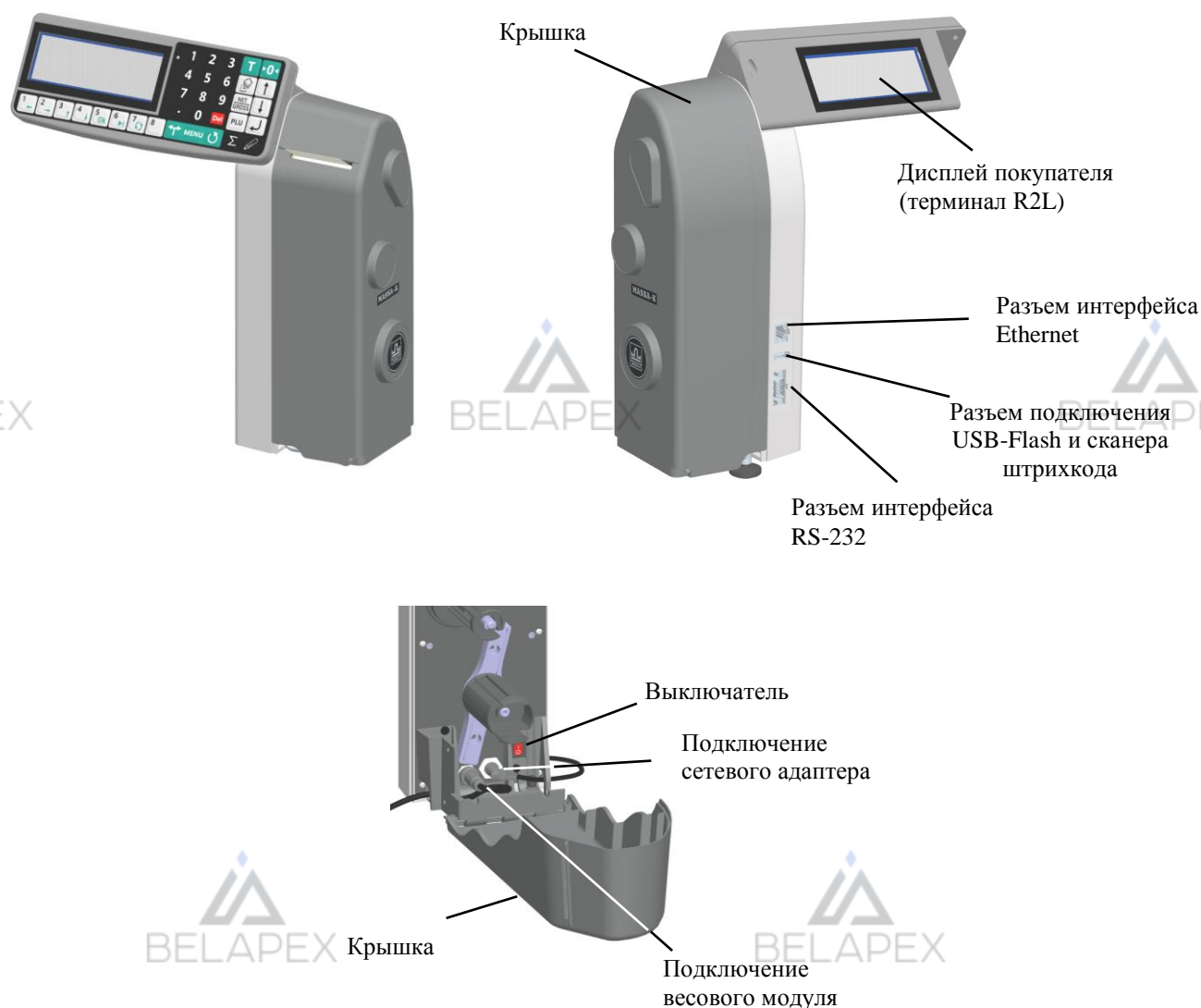
Рис. 2.1 – Общий вид терминалов RL и R2L
