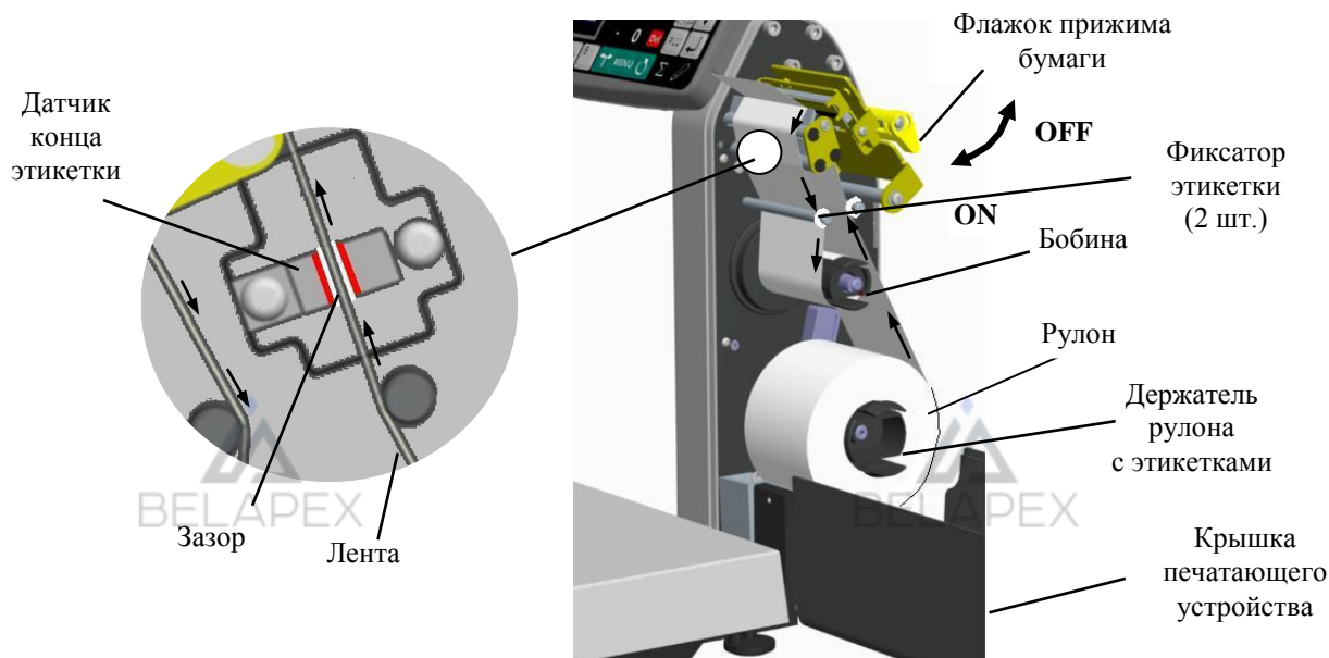
Рис. 2.6 – Установка рулона в терминалы RL и R2L
