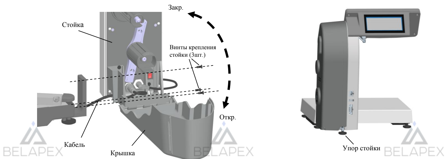
Рис. 2.3 – Крепление терминалов в весах МК-RL, МК-R2L
