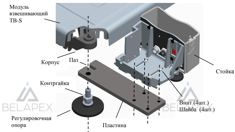
Рис. 2.4 – Крепление терминалов к модулю взвешивающему ТВ
